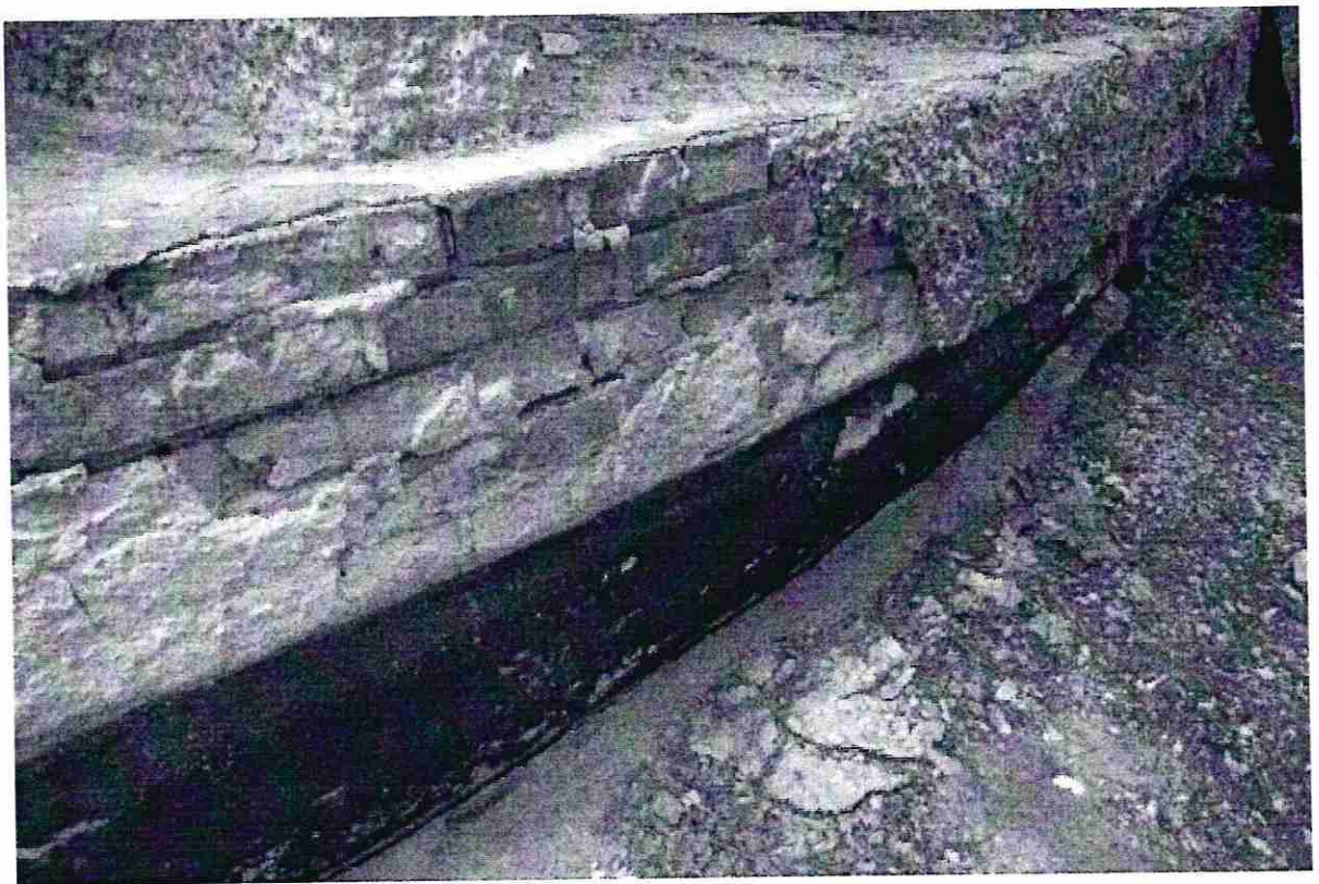
Рис. 6. Фундамент. На основе фото 2025 г.
