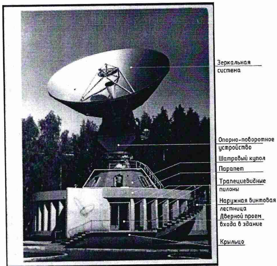
Рис. 2. Схема архитектурно-художественного оформления главного фасада. На основе фото 1967 года.
