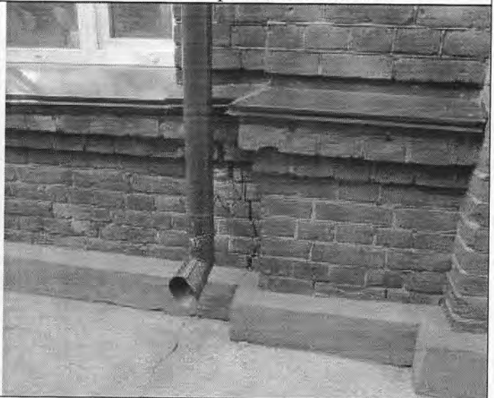
22. Деформационная трещина в стене северо-восточного фасада и отмостке
