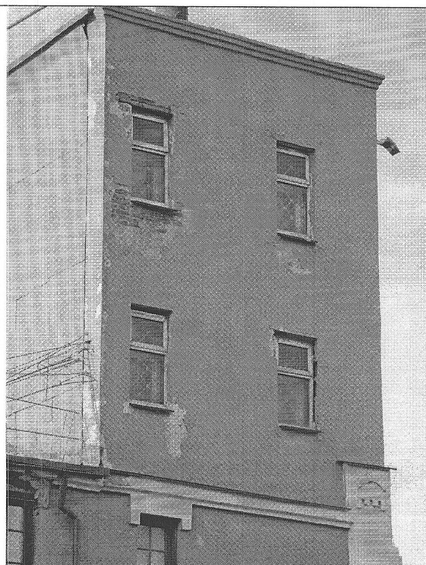
7. Дефекты отделки стены 4 и 5 этажей северо-восточного (главного) фасада.
