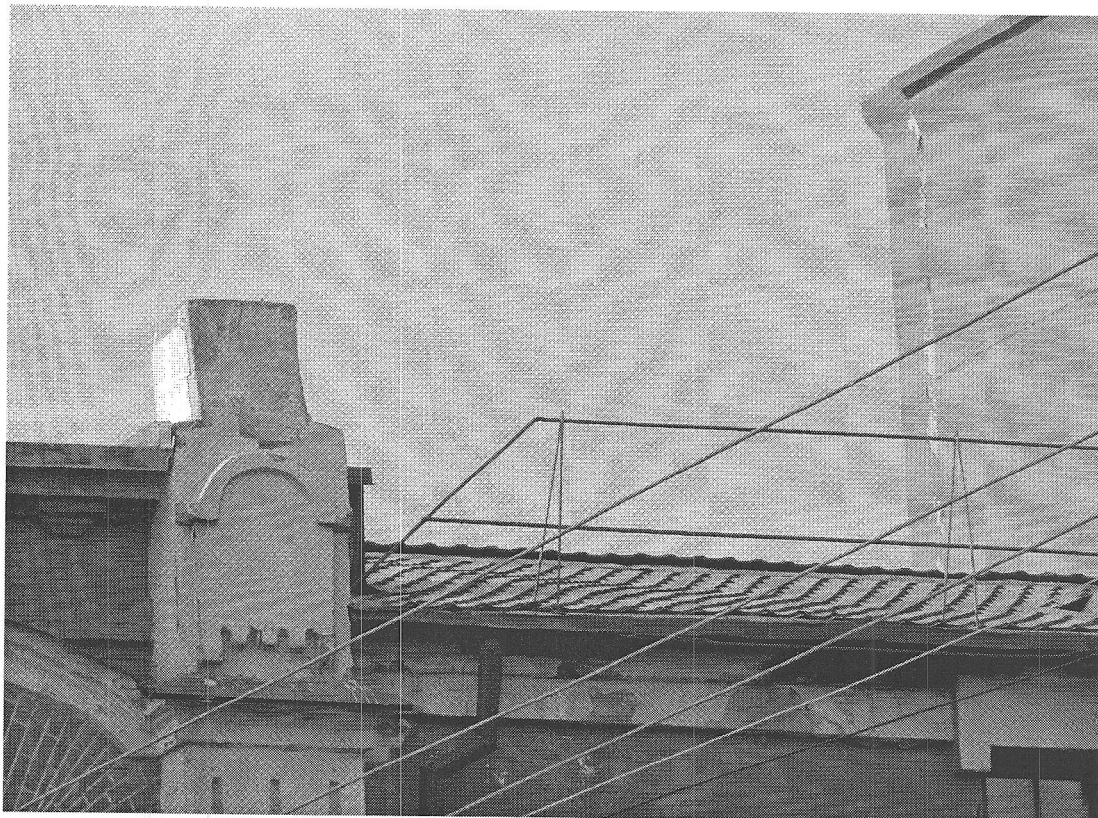
9. Дефекты отделочного слоя декоративных элементов и карниза. Фрагмент кровли.
