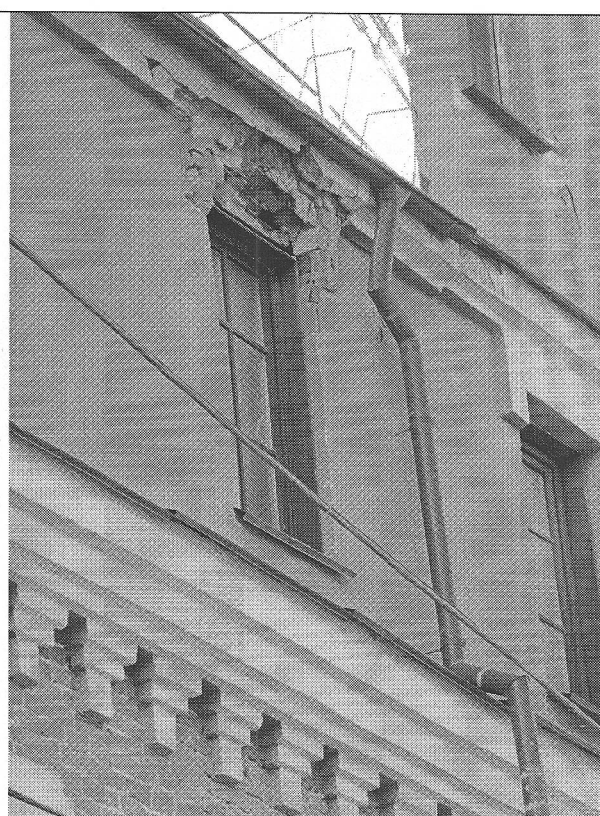
8. Разрушение надоконной перемычки и декоративного элемента окна. Фрагмент декоративного оформления междуэтажного карниза.
