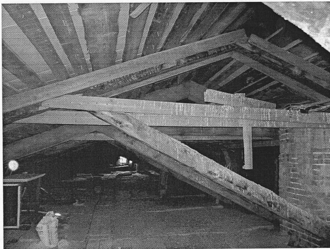
10. Конструкции крыши.
