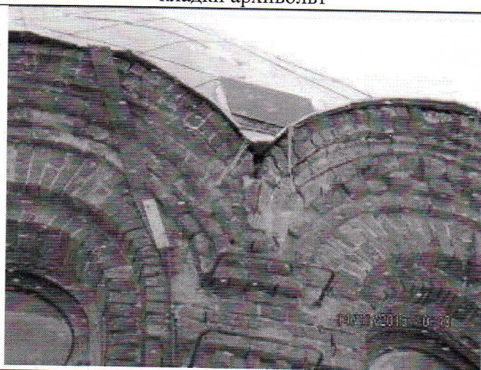
21. Выветривание раствора в швах кирпичной кладки архивольта
