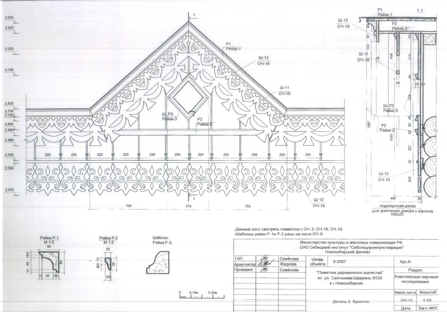
Оформление щипца. Слуховое окно. Подзоры, рейки. Чертеж от 08.2007 г.
