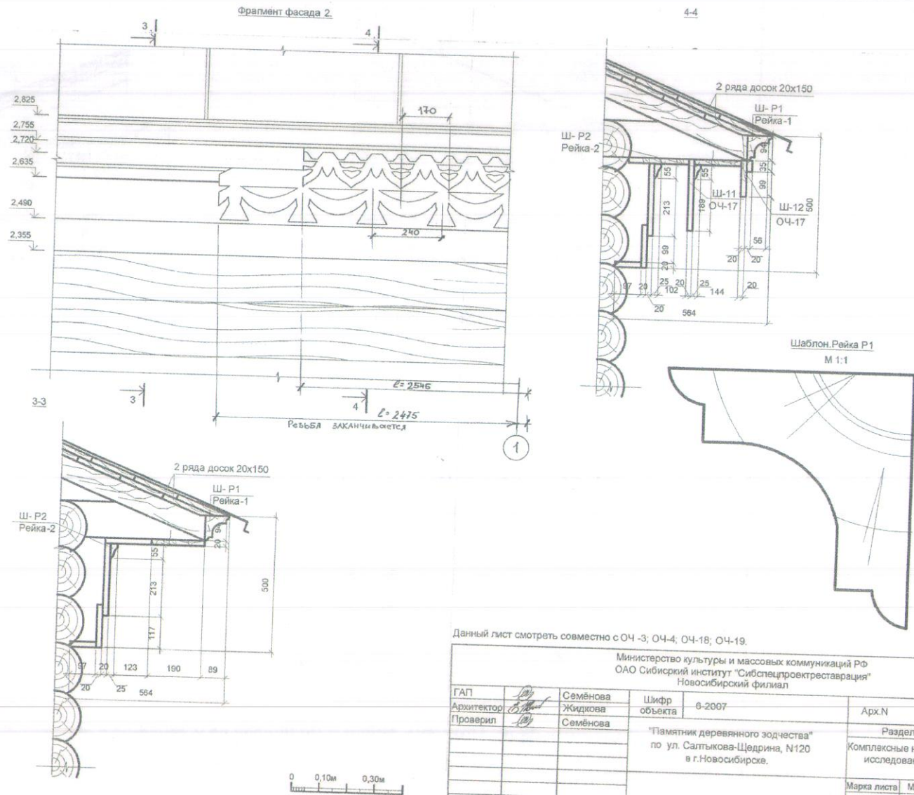
Венчающие карниз и фриз. Подзоры, рейки и подшивка северо-западного фасада. Чертеж от 08.2007 г. ОЧ-9.
