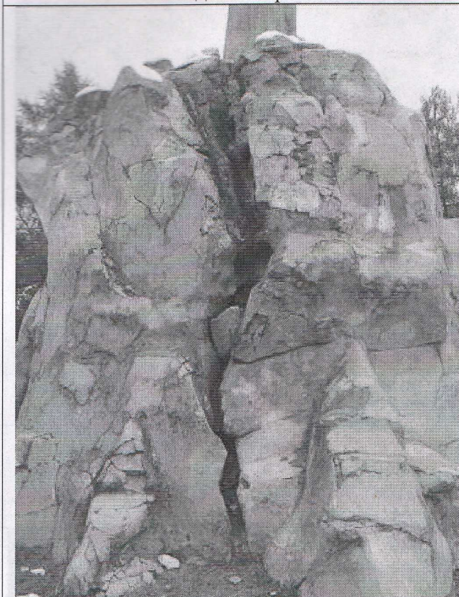
9. Дефекты покрытия монумента, северо-западная сторона
